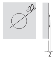
せり防止突起詳細図
