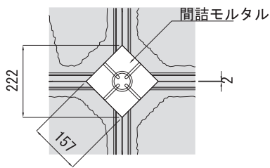
連結部詳細図
