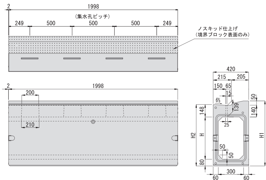
水路幅300 単位(mm)
