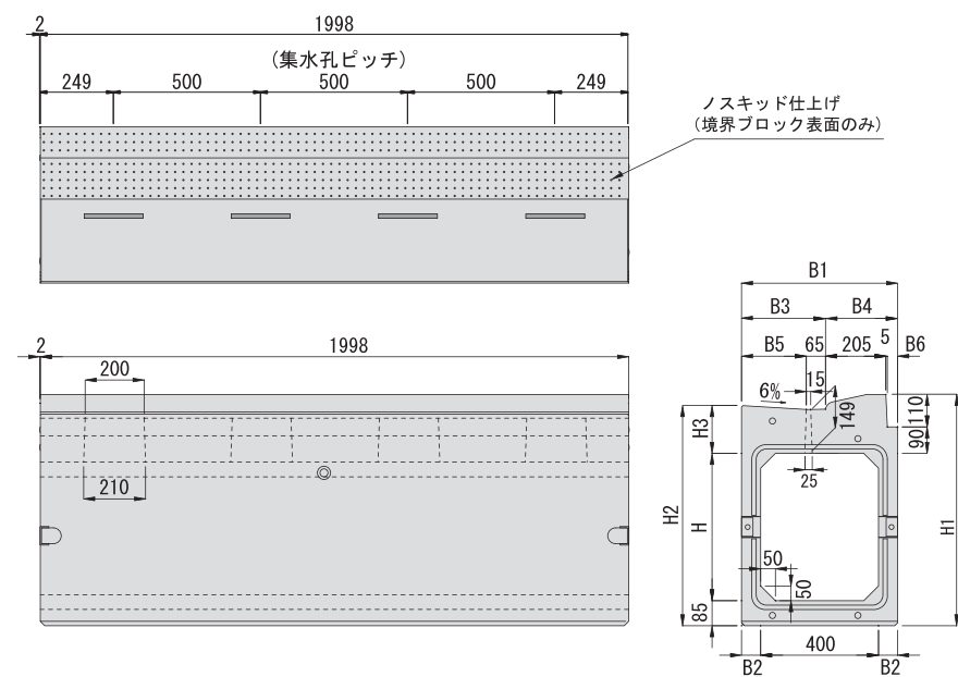
水路幅400 単位(mm)
