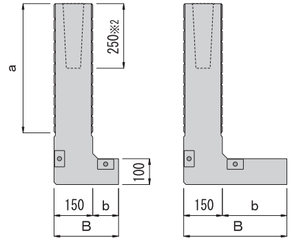
土留めタイプ 底版 (B=400・450※1)
