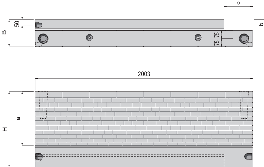
底版 (B=250)
